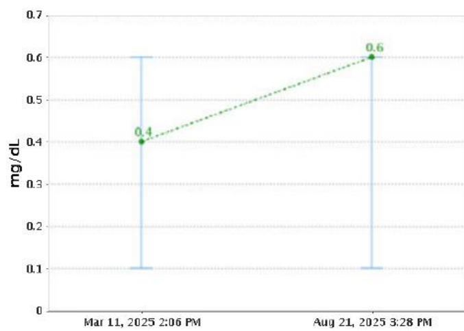
Total Bilirubin
